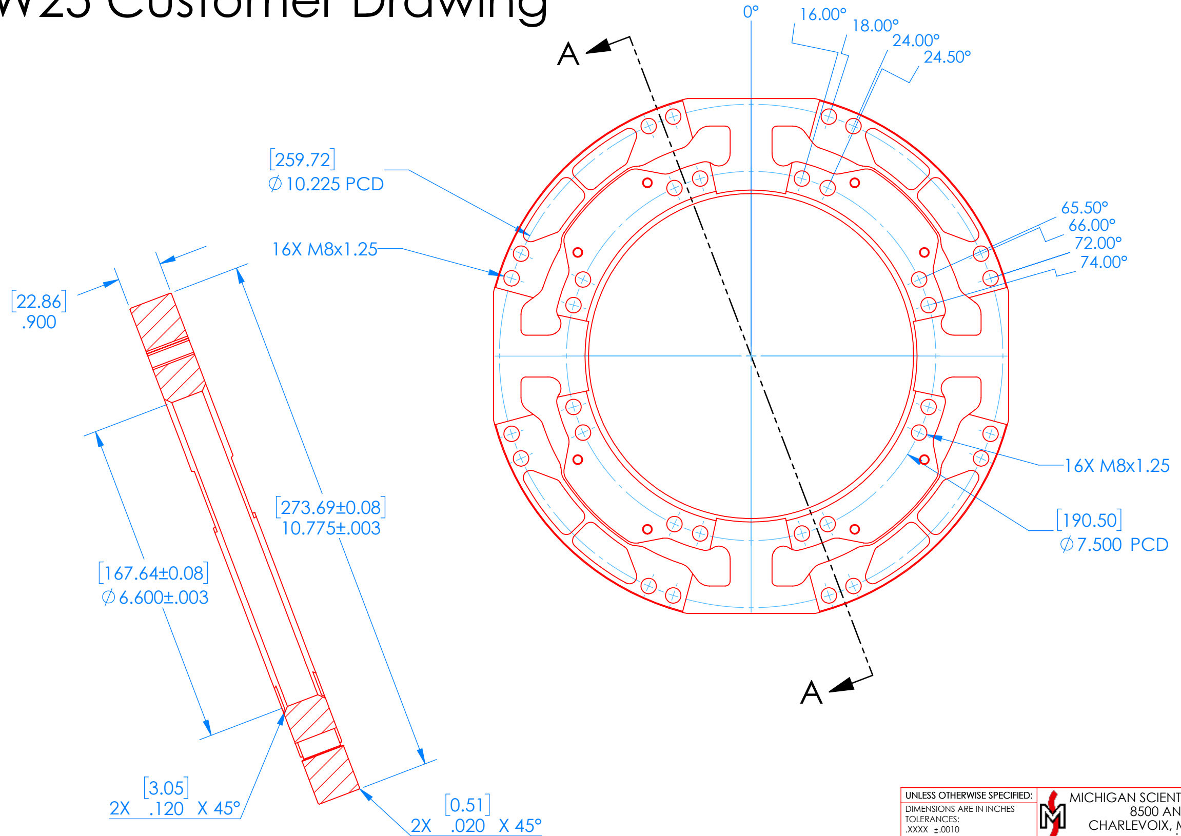
SECTION A-A
