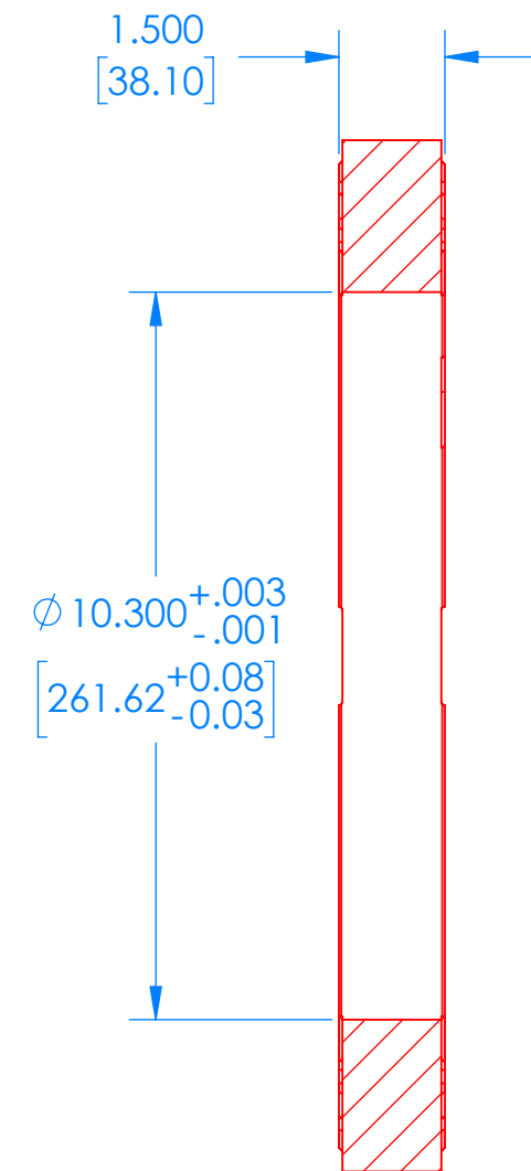
SECTION A-A
